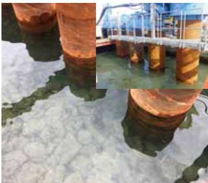
捨石貫入状況
