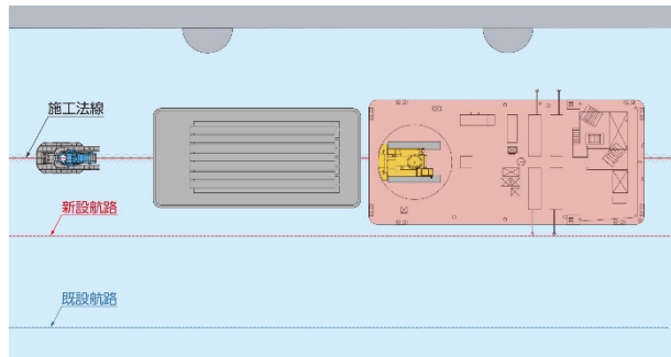
退避時配置図
